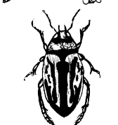
Vabalai Coleoptera
